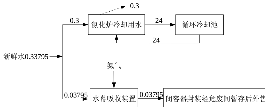
图1 本项目水平衡图 单位: \text{m}^3/\text{d}
