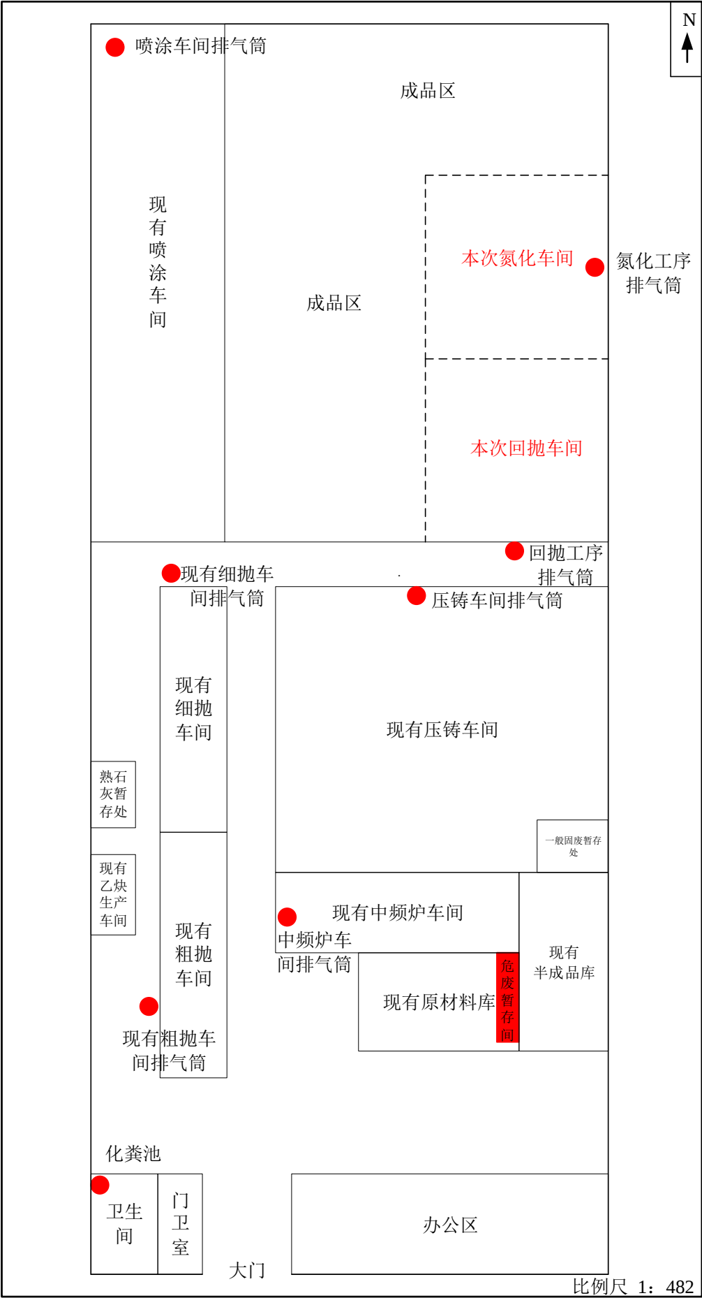
附图三 本项目厂区平面布置示意图
