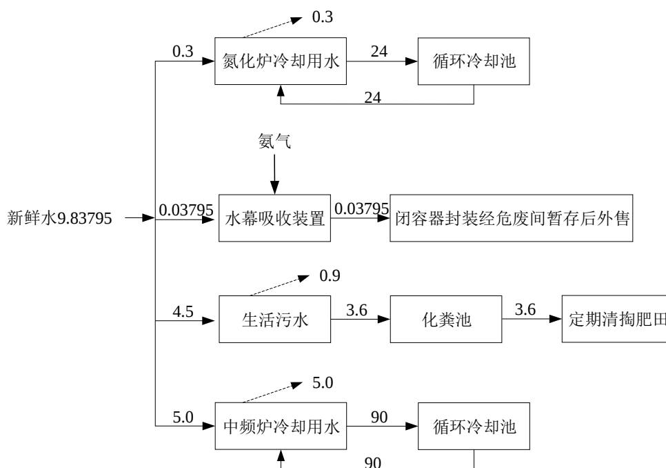
图2 本项目建成后全厂水平衡图 单位: \text{m}^3/\text{d}
