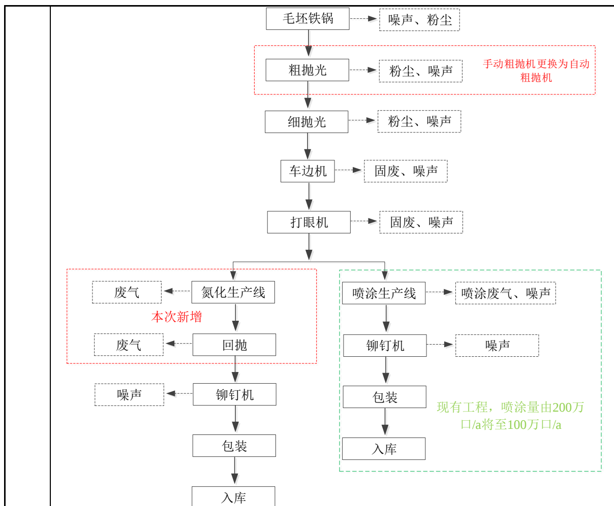
图3 项目总体工艺流程意图
