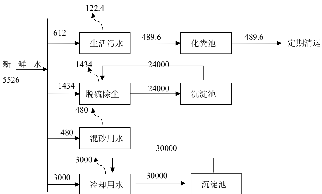
图 2-3 项目改建完成后水平衡图 单位：m 3 /a
