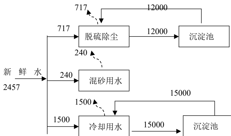
图 2-2 改建项目置换工程水平衡图 单位：m 3 /a
