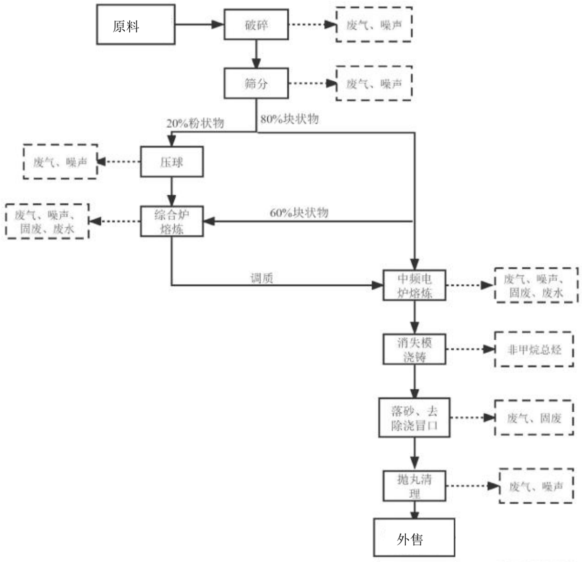
图 2-6 改建项目置换工程生产工艺流程及排污节点图
