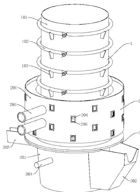
图 4-1 综合利用环保节能炉熔炼结构图
