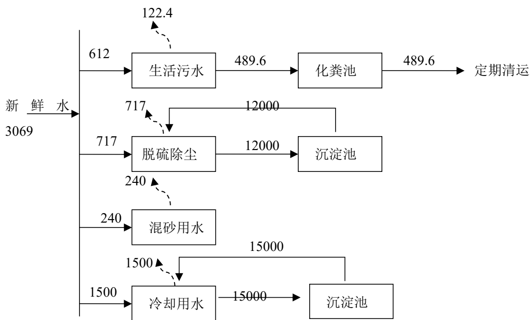
图 2-1 项目现有工程水平衡图 单位：m³/a
