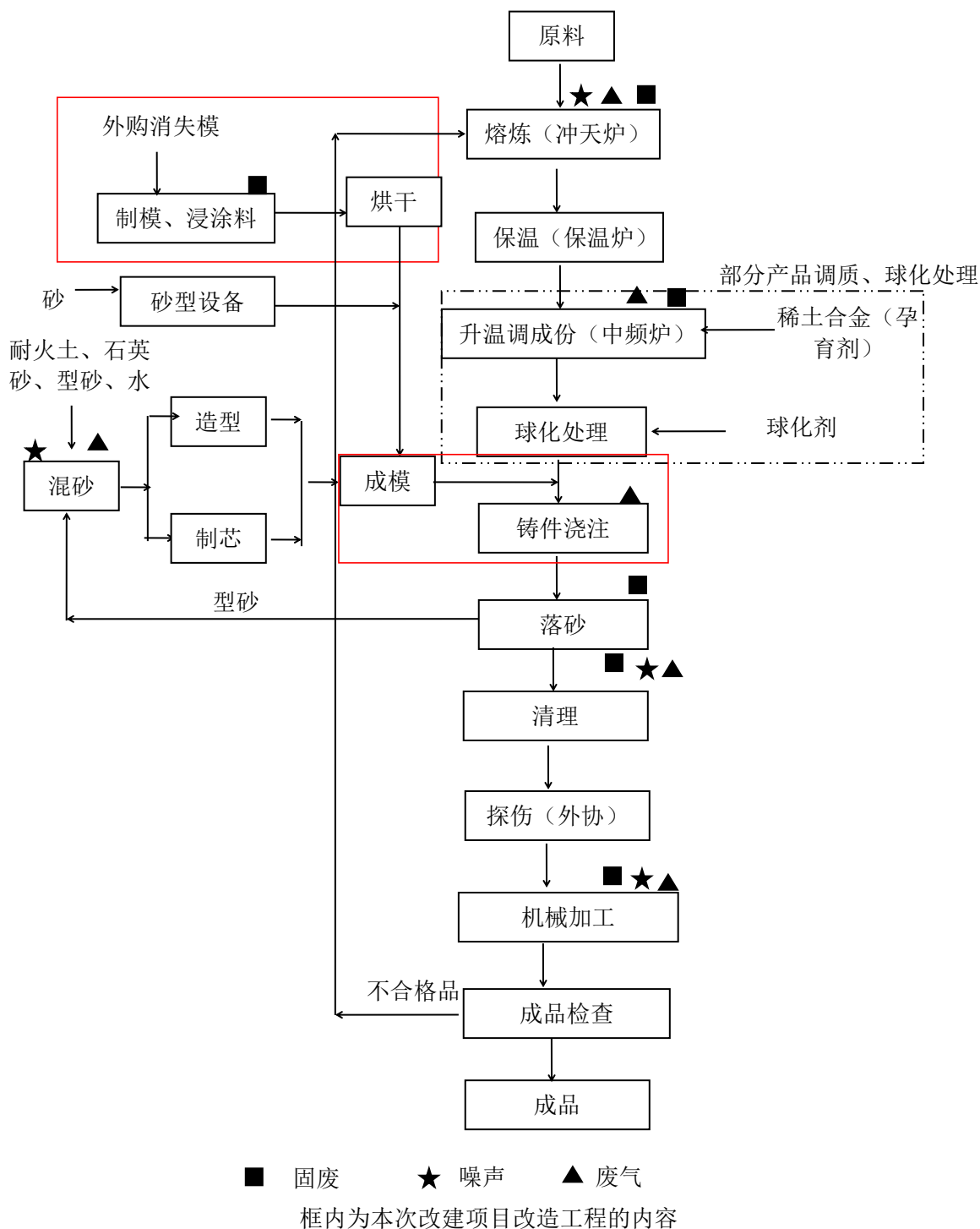
图 2-4 改建项目改造工程生产工艺流程及排污节点图
