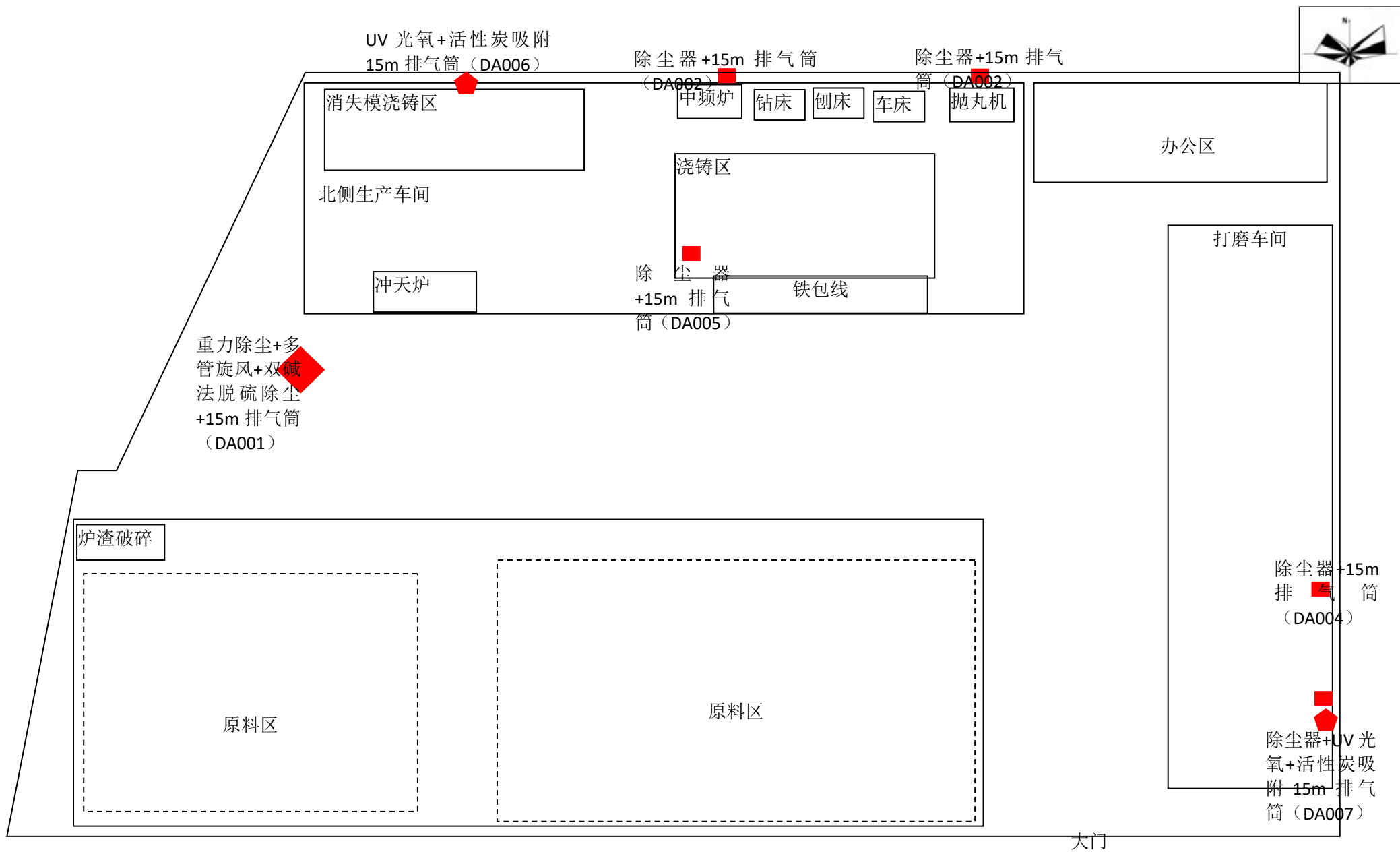
附图三 厂区平面布置图
