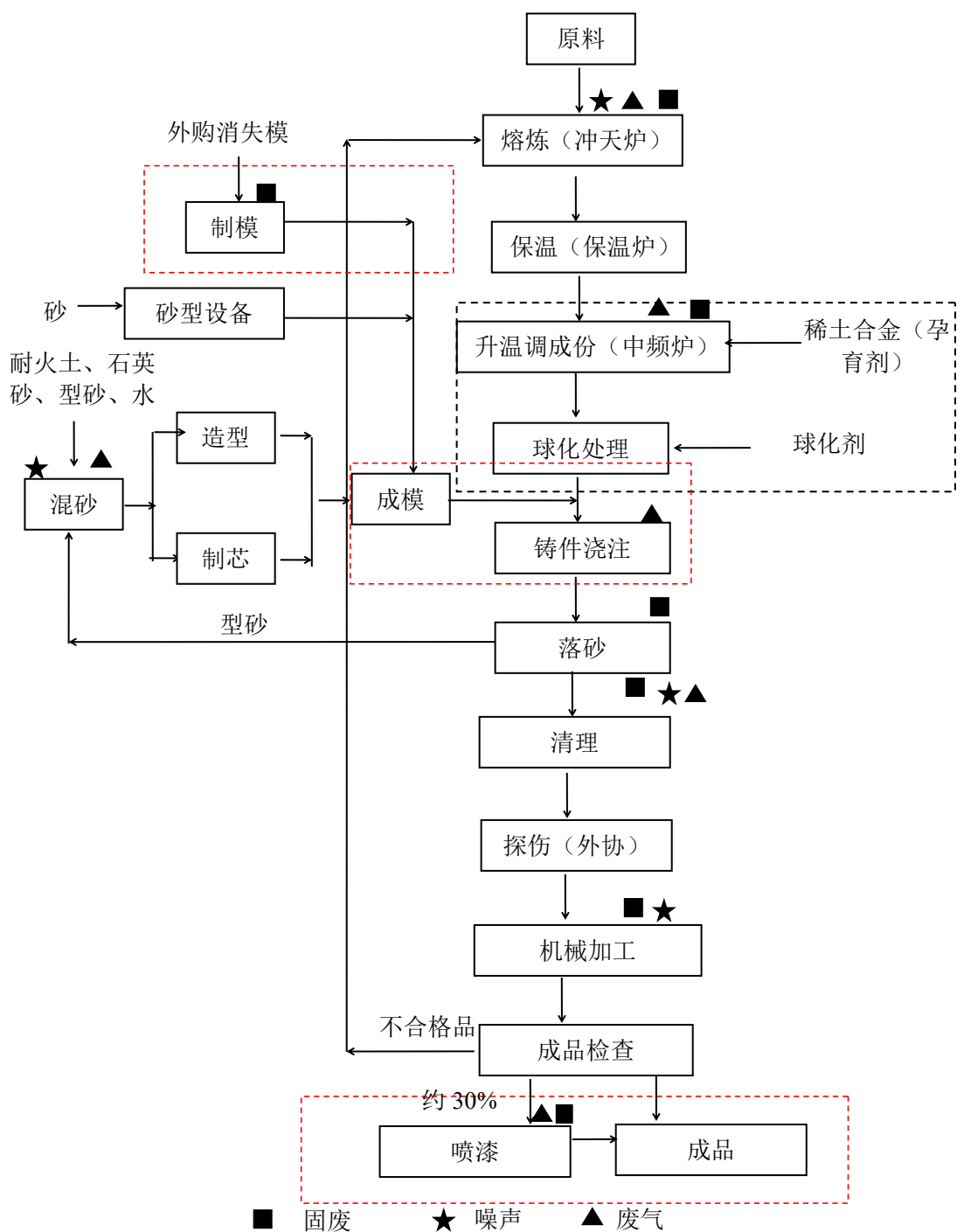
图 2-2 生产工艺流程及排污节点图
