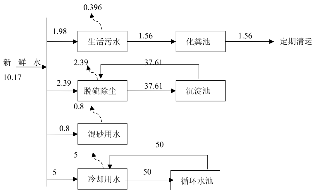
图 2-1 项目改建完成后水平衡图 单位: m³/d
