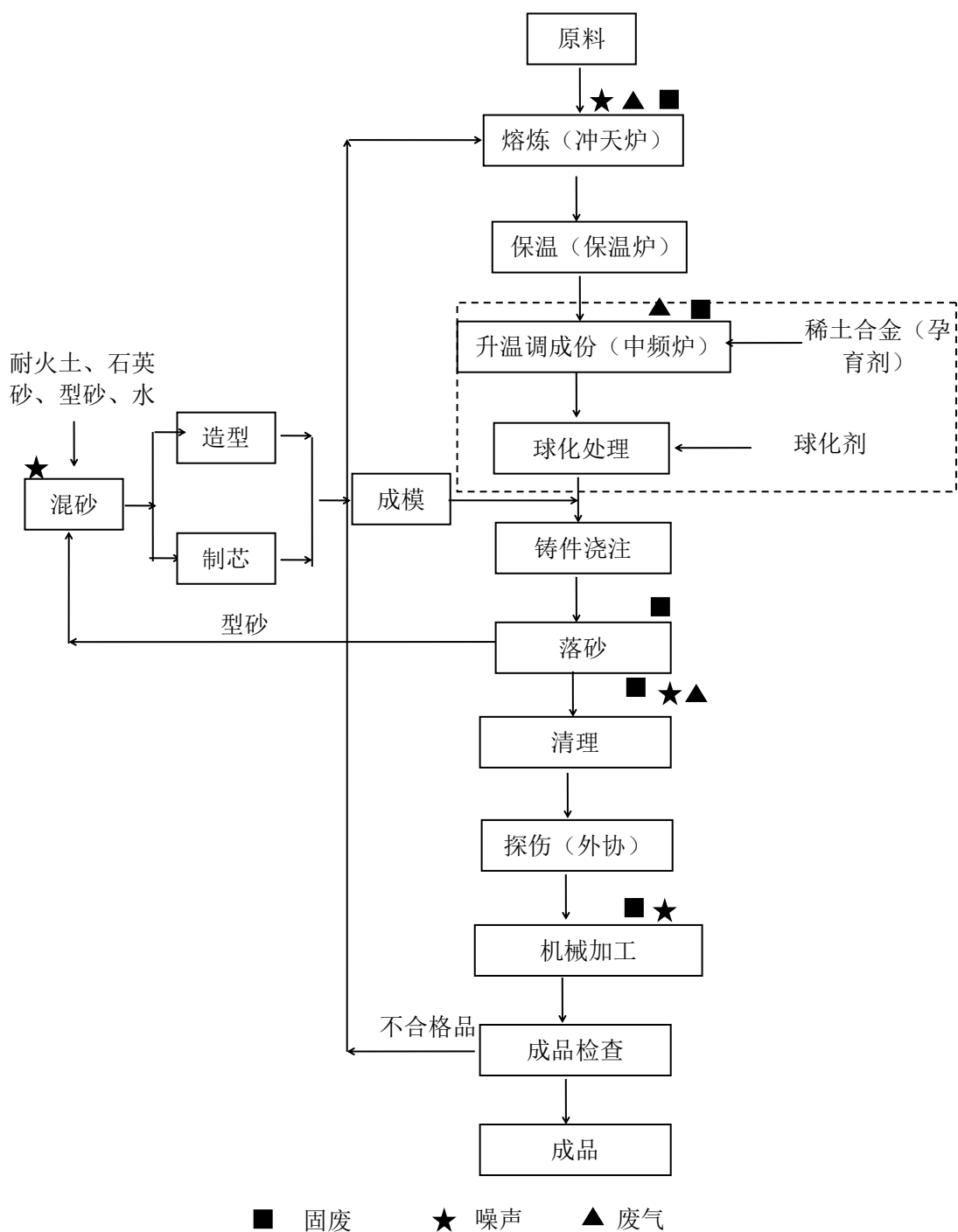
图 2-4 铸件生产工艺流程及排污节点图
